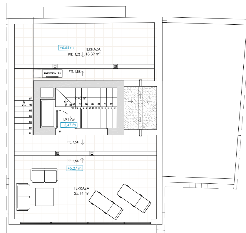
PLANTA TORRETA
