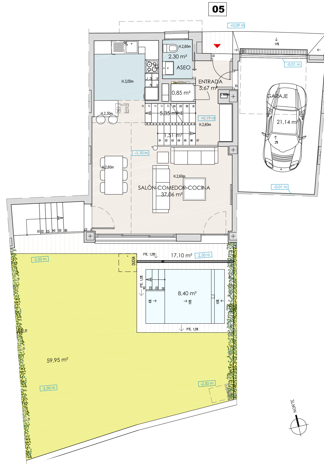
PLANTA BAJA
