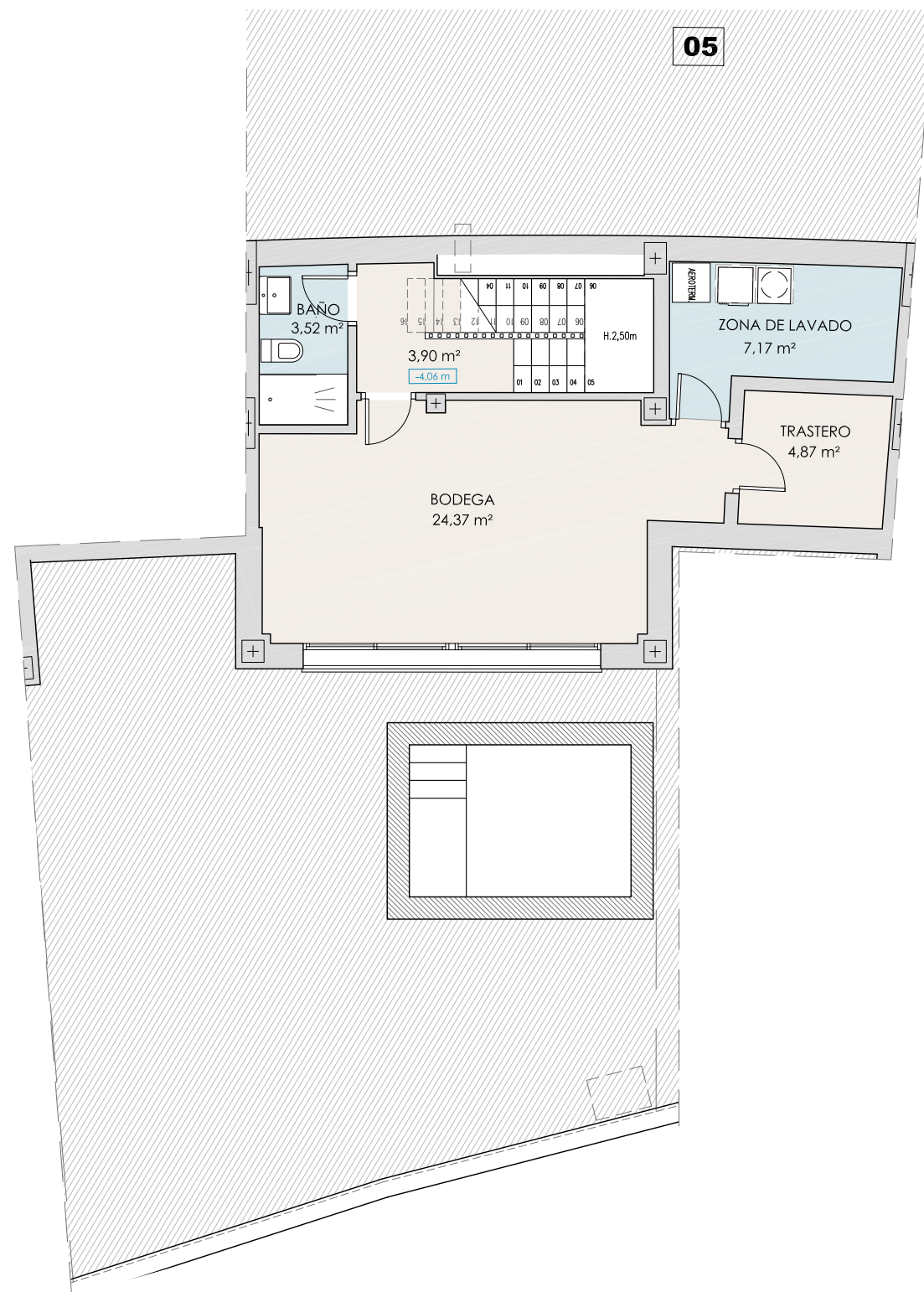
PLANTA SEMISÓTANO
