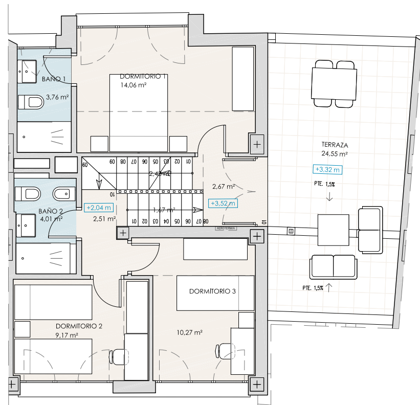
PLANTA PRIMERA
