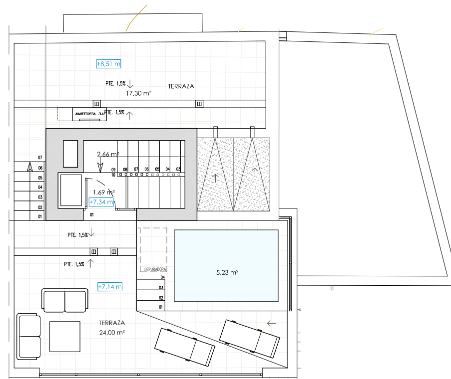
PLANTA TORRETA
