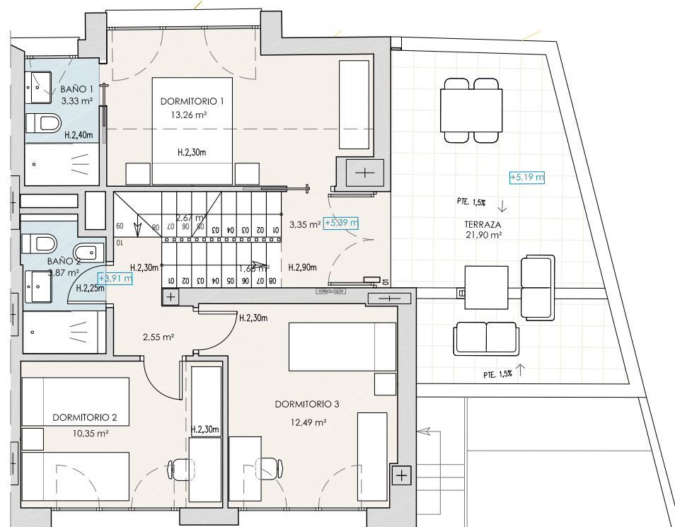
PLANTA PRIMERA
